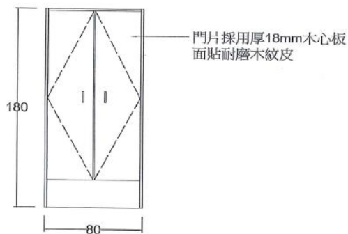
衣櫃立面圖
