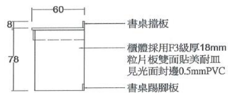
書桌側視圖
